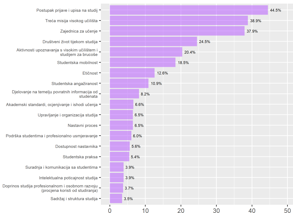
Slika 3: Aspekti studentskog iskustva koje studenti smatraju najmanje važnim za ukupno zadovoljstvo studiranjem
